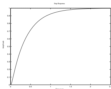
Abb. 11.25: MATLAB-Grafik der Führungsübergangsfunktion des geregelten Gleichstrommotors
