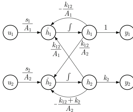
Abb. 4.14: Signalflussgraf des Modells (4.50), (4.51)
