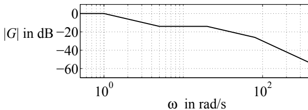
Abb. 6.54: Geradenapproximation eines Amplitudenganges
