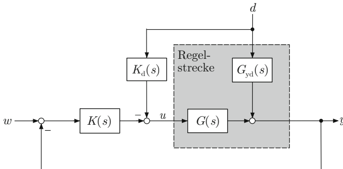
Abb. 13.1: Blockschaltbild einer Störgrößenaufschaltung
