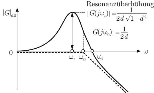
Abb. 6.40: Resonanzüberhöhung beim PT_2 -Glied für 0 < d < \frac{1}{\sqrt{2}}
