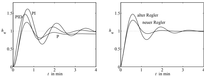
Abb. 9.3: Führungsübergangsfunktion des Temperaturregelkreises für unterschiedliche Reglertypen (links) und für PID-Regler mit unterschiedlicher Nachstellzeit T_I (rechts)
