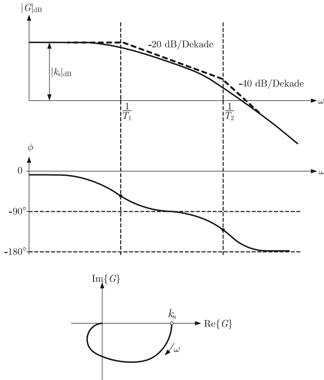
Abb. 6.33: Bodediagramm und Ortskurve des PT 2 -Gliedes (6.111)
