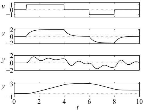
Abb. 5.44: Verlauf der Eingangs- und Ausgangsgrößen einfacher Übertragungsglieder
