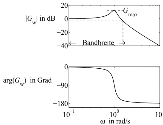
Abb. 7.3: Bodediagramm des Führungsfrequenzganges mit Kennzeichnung wichtiger Kennwerte
