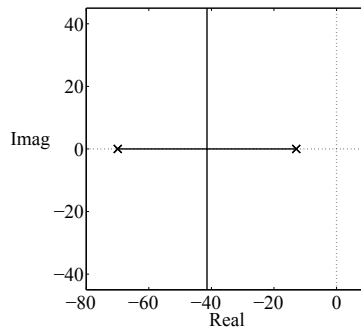
Abb. A.53: Wurzelortskurve des P-geregelten Gleichstrommotors
