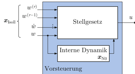
Abb. 7.23: Struktur der Vorsteuerung (7.64)
