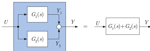
Abb. 6.23: Parallelschaltung zweier Übertragungsglieder
