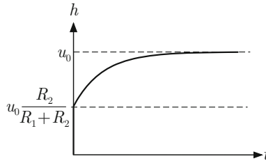
Abb. A.26: Übergangsfunktion des RC-Gliedes
