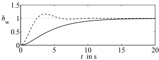
Abb. 7.14: Führungsübergangsfunktion des Regelkreises
