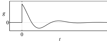
Abb. 5.19: Gewichtsfunction eines Systems zweiter Ordnung
