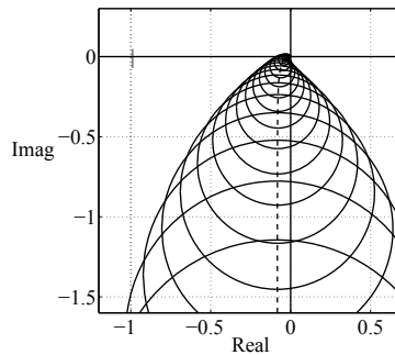
Abb. 8.26: Toleranzband für die Ortskurve der offenen Kette des Motorregelkreises
