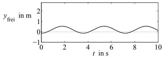
Abb. 5.6: Eigenbewegung der Verladebrücke
