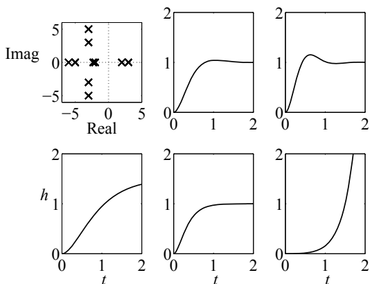
Abb. 6.45: PN-Bild und Übergangsfunktionen von PT_2 -Gliedern
