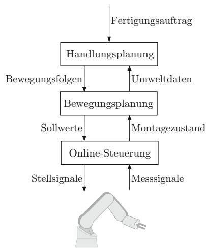
Abb. 2.7: Hierarchische Struktur von Robotersteuerungen
