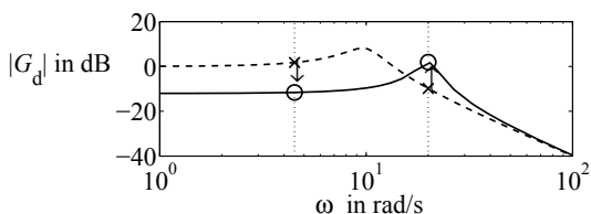
Abb. 7.19: Verschiebung der Störübertragungsfunktion durch die Regelung
