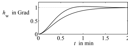
Abb. 12.3: Führungsübergangsfunktionen der entworfenen Temperaturregelkreise
