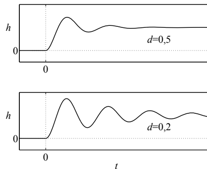
Abb. 5.33: Übergangsfunktionen von PT_2 -Gliedern mit kleiner Dämpfung
