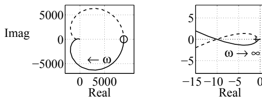
Abb. 8.11: Ortskurve einer offenen Kette siebenter Ordnung (Gesamtbild (links) und Ausschnitt (rechts))
