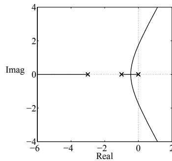
Abb. A.55: Wurzelortskurve für das P-geregelte System
