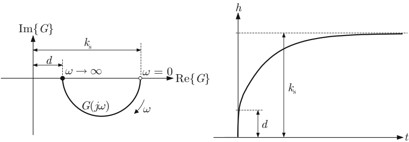
Abb. 6.29: Zusammenhang zwischen Frequenzgang G(j\omega) und Übergangsfunktion h(t)
