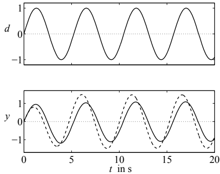
Abb. 7.16: Verhalten des Regelkreises bei sinusförmiger Störung für T_I = 5 \text{ s} (—) und T_I = 1 \text{ s} (---)
