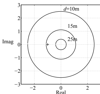
Abb. A.46: Ortskurve der offenen Kette der Lautsprecheranlage für unterschiedliche Mikrofon-Lautsprecher-Entfernungen
