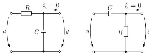
Abb. 5.43: RC-Glieder
