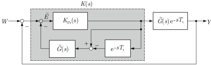
Abb. 12.9: Smithprädiktor
