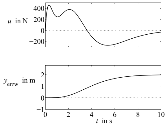
Abb. 5.7: Erzwungene Bewegung der Verladebrücke
