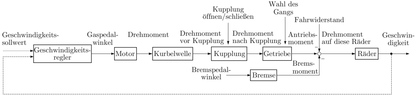
Abb. A.3: Blockschaltbild des Antriebsstranges
