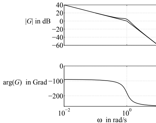
Abb. A.29: Geradenapproximation des hydraulischen Stellantriebs
