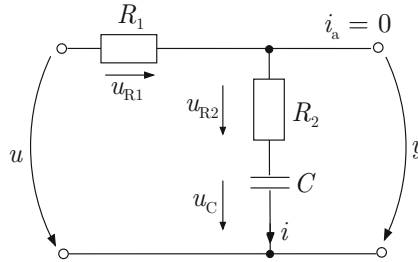
Abb. A.13: RC-Glied
