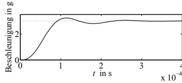
Abb. A.85: Messergebnis bei Beschleunigung 3g
