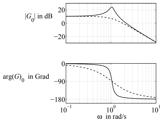
Abb. A.71: Bodediagramm des unregelmäßig (—) und des stabilisierten Schiffes (---)
