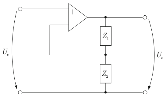
Abb. 6.27: Operationsverstärker mit Beschaltung
