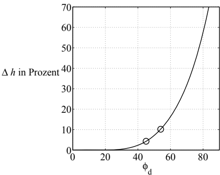
Abb. 10.5: Abhängigkeit der Überschwingweite \Delta h vom Winkel \phi_d
