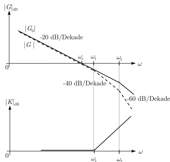
Abb. 11.15: Verbesserung des Übergangsverhaltens durch Verwendung eines PD-Reglers
