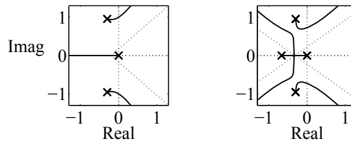
Abb. A.58: Wurzelortskurve des Hydraulikantriebs mit P-Regler (links) und PT_1 -Regler (rechts)
