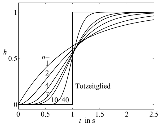
Abb. 6.69: Übergangsfunktion von PT n -Näherungen des Totzeitgliedes mit T_t = 1 s
