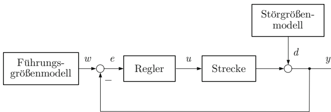
Abb. 7.7: Standardregelkreis mit Führungsgrößenmodell und Störgrößenmodell
