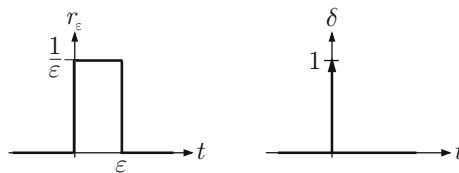
Abb. 5.18: Definition und Darstellung des Diracimpulses
