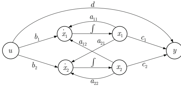
Abb. 4.8: Signalflussgraph eines Systems zweiter Ordnung
