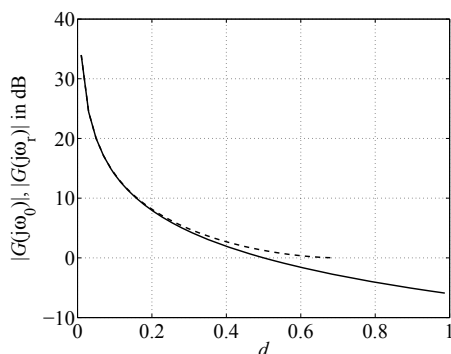
Abb. 6.43: Abhängigkeit von |G(j\omega_r)| - - - und |G(j\omega_0)| — von der Dämpfung d (bei |k_s| = 1 )
