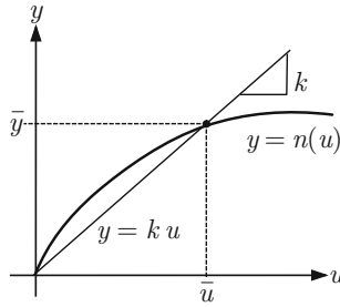
Abb. 4.24: Linearisierung der TORICELLI-Gleichung
