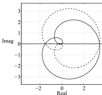
Abb. A.48: Ortskurve der D-Kette
