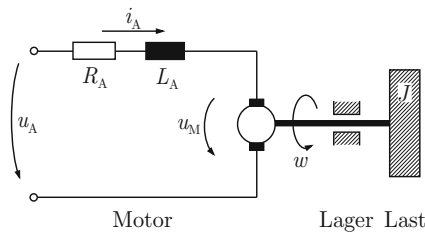
Abb. 5.12: Gleichstrommotor
