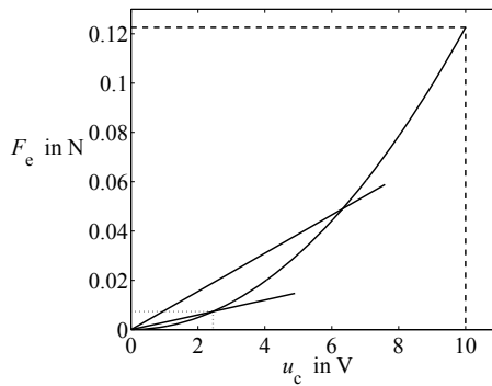
Abb. A.83: Linearisierung des nichtlinearen Zusammenhanges zwischen u_c und F_e
