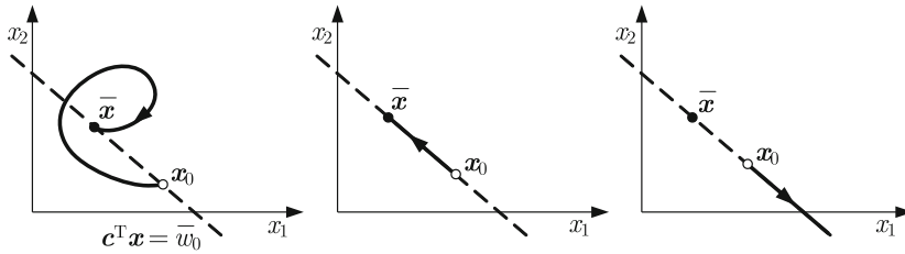
Abb. 6.62: Umsteuerung von Systemen mit stabiler und instabiler interner Dynamik
