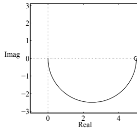
Abb. 6.73: Ortskurve des Raumes
