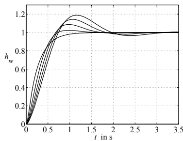
Abb. 8.27: Schar der Führungsübergangsfunktionen des geregelten Motors bei J = 0,1, \dots, 0,5
