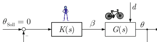
Abb. A.59: Fahrrad als Regelstrecke
