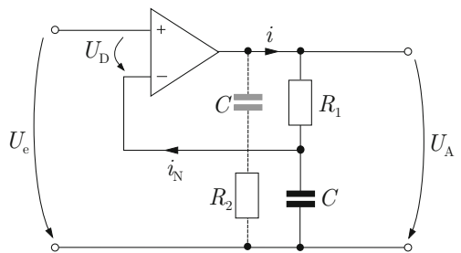
Abb. A.28: Beschaltung des Operationsverstärkers mit dynamischen Elementen
