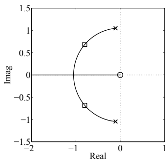
Abb. A.69: Wurzelortskurve des Stabilisatorregelkreises (Pole \square bei k = 0,35 )
