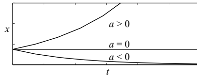
Abb. 5.1: Eigenbewegung eines Systems erster Ordnung für x_0 = 1
