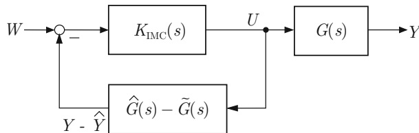
Abb. 12.16: Smithprädiktor-Regelkreis mit Modellunsicherheiten
