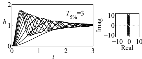
Abb. 10.7: Übergangsfunktion eines Schwingungsgliedes mit Polen bei \delta_e = 1 und \omega_e = 1, \dots, 10
