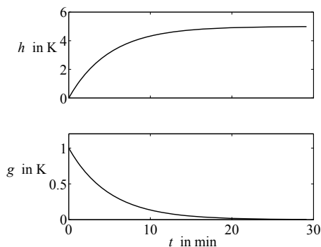
Abb. 5.51: Übergangsfunktion und Gewichtsfunktion eines Raumes
