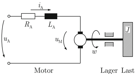
Abb. A4.1: Gleichstrommotor
