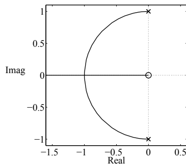
Abb. A.66: Wurzelortskurve zur Bestimmung des kritischen Widerstandes
