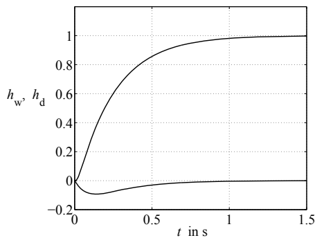
Abb. 11.24: Führungsübergangsfunktion und Störübergangsfunktion des geregelten Gleichstrommotors
