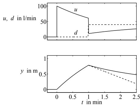
Abb. 1.11: Störverhalten des Behälters
