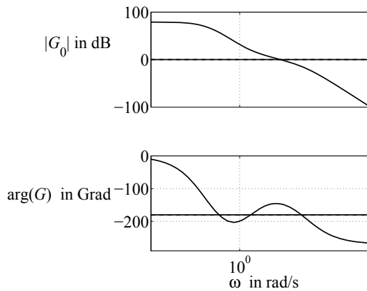
Abb. 8.18: Bodediagramm eines Systems mit positivem Phasenrand
