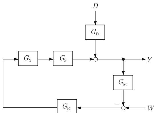
Abb. 6.26: Blockschaltbild eines Regelkreises
