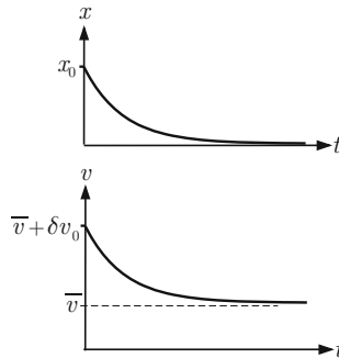
Abb. A.16: Eigenbewegung des Fahrzeugs
