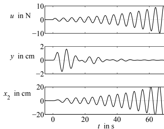
Abb. 5.25: Eingangsgröße, Ausgangsgröße und Position der Masse m_1 bei Erregung durch u(t) = e^{0,0344t} \sin 1,206 t
