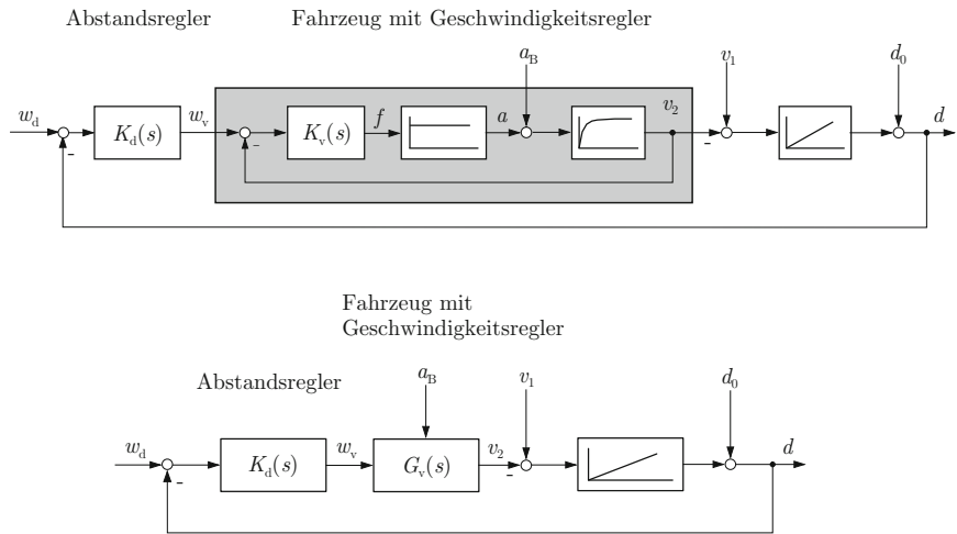
Abb. A.81: Kaskadenregelung des Fahrzeugabstandes
