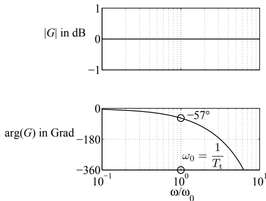
Abb. 6.67: Bodediagramm des Totzeitgliedes
