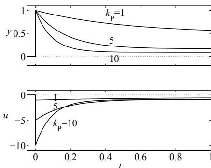
Abb. 7.10: Störübergangsfunktion eines Regelkreises mit Proportionalregler ( k_P = 1, 5 und 10 )
