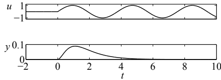
Abb. 6.20: Eingangsgröße und Ausgangsgröße des in Aufgabe 6.8 betrachteten Systems
