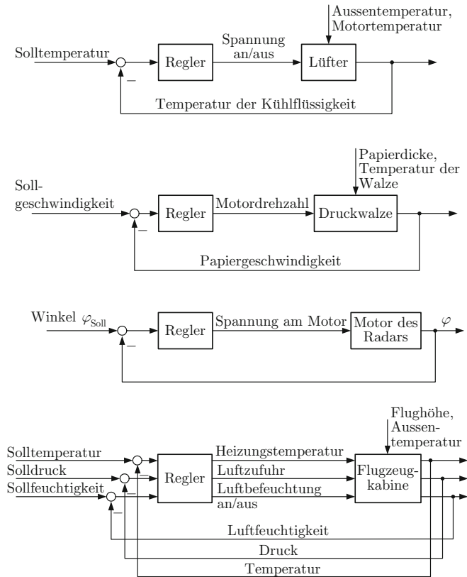
Abb. A.1: Blockschaltbilder der Regelkreise
