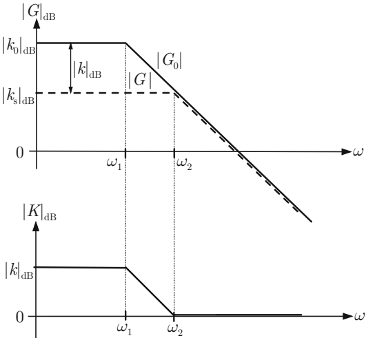
Abb. 11.12: Verbesserung des statischen Verhaltens mit Hilfe eines integrierenden Korrekturgliedes
