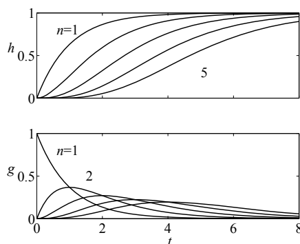
Abb. 5.34: Übergangsfunktionen und Gewichtsfunktionen von PT_n -Gliedern ( n = 1, 2, \dots, 5 )
