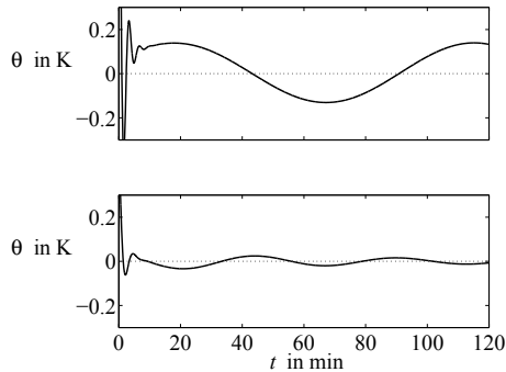
Abb. A.52: Sekundärlufttemperatur bei impulsförmiger Erregung (oben: unregelt; unten: mit Sekundärlufttemperaturregelung)
