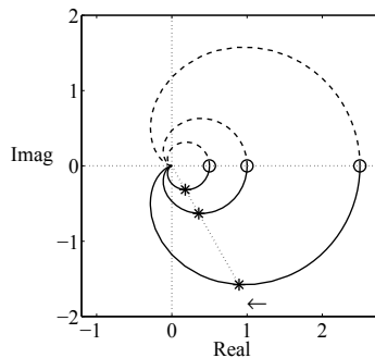
Abb. A.38: Ortskurve der Regelstrecke für k = 1, 2 und 5
