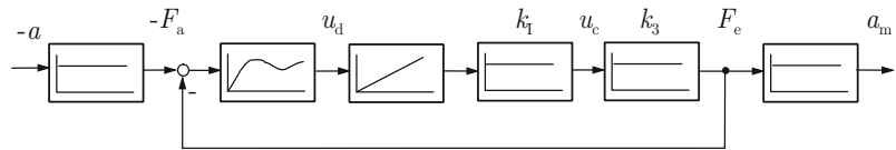
Abb. A.82: Umgezeichnetes Blockschaltbild des Sensors
