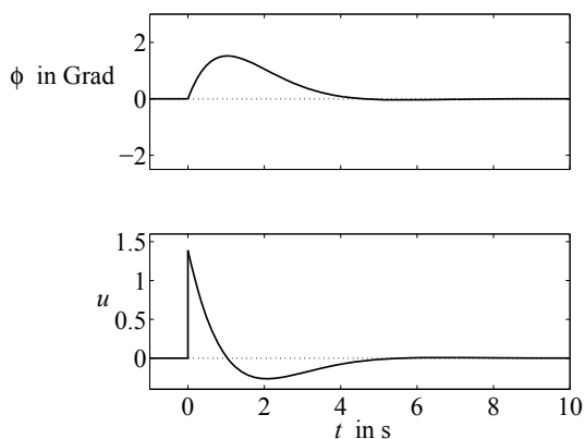
Abb. A.70: Bewegung des stabilisierten Schiffes bei impulsförmiger Anregung
