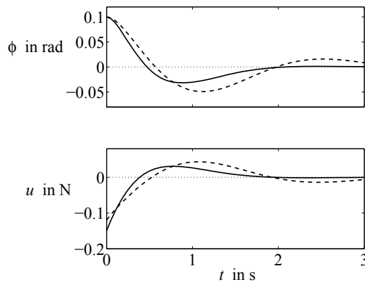
Abb. 10.19: Eigenbewegung des Regelkreises bei \phi(0) = 0,1 rad
