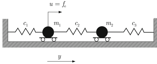
Abb. 4.17: Gekoppeltes Feder-Masse-System
