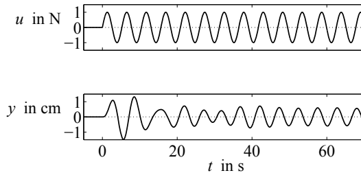
Abb. 5.26: Verhalten des Feder-Masse-Dämpfer-Systems bei sinusförmiger Erregung u(t) = \sin 1,206 t
