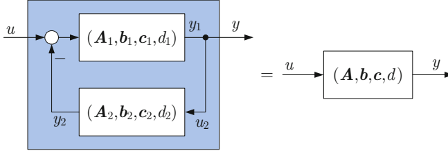
Abb. 4.20: Rückkopplungsschaltung zweier Teilsysteme
