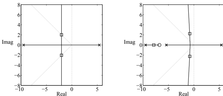
Abb. 10.18: Wurzelortskurve bei genauer (links) und ungenauer (rechts) Kompensation des Regelstreckenpols durch die Nullstelle des Reglers
