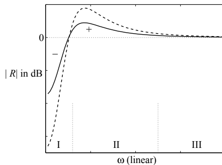
Abb. 7.12: Typischer Verlauf des Betrages des Regelfaktors R(j\omega)
