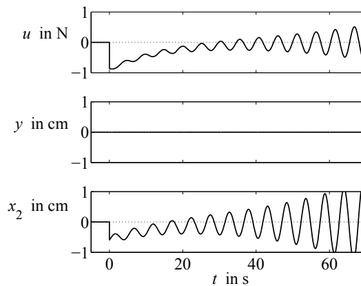
Abb. 5.28: Verhalten des Feder-Masse-Dämpfer-Systems für ein vom Eingangsgrößengenerator erzeugtes Signal u(t)
