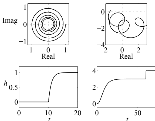
Abb. 6.68: Ortskurven und Übergangsfunktionen zweier totzeitbehafteter Systeme
