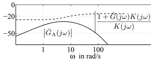
Abb. 8.25: Prüfung der Stabilitätsbedingung (8.52)
