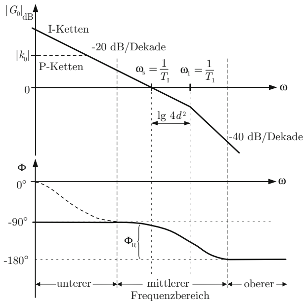
Abb. 11.1: Bodediagramm der offenen Kette
