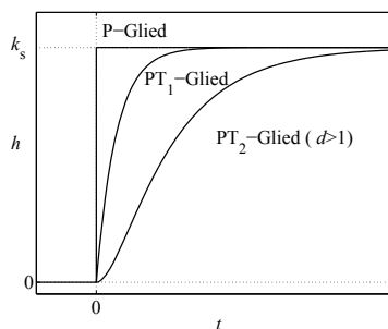
Abb. 5.30: Übergangsfunktion von P-Gliedern
