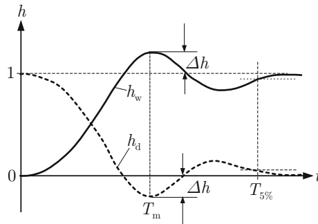
Abb. 7.2: Übergangsfunktionen bei sprungförmiger Störung bzw. Führung
