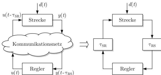
Abb. 8.15: Realisierung einer Regelung mit Hilfe eines digitalen Kommunikationsnetzes
