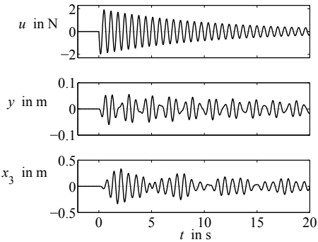
Abb. A.35: Verhalten des Hochhauses bei sinusförmiger Erregung
