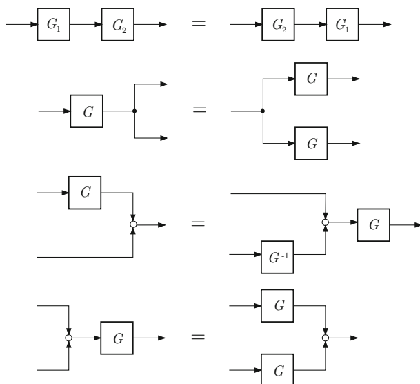
Abb. 6.25: Weitere Regeln für das Umformen von Blockschaltbildern
