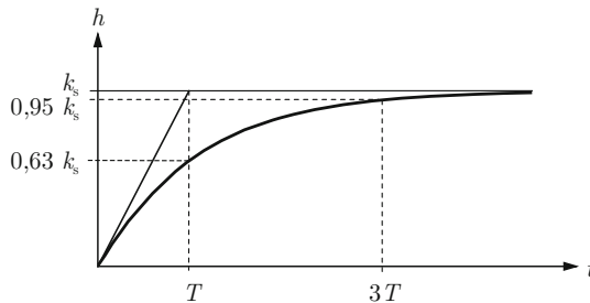
Abb. 5.47: Übergangsfunktion eines PT_1 -Gliedes
