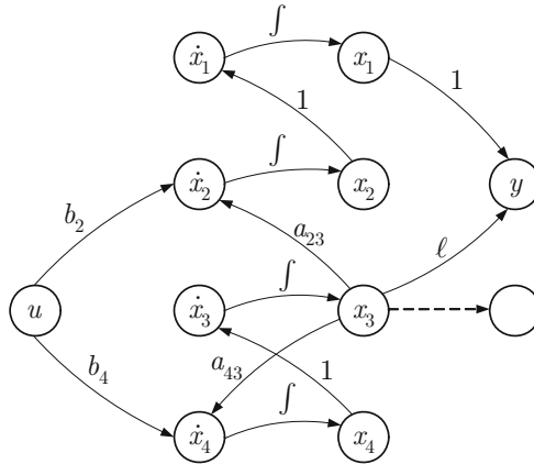
Abb. A.27: Signalflussgraf der Verladebrücke
