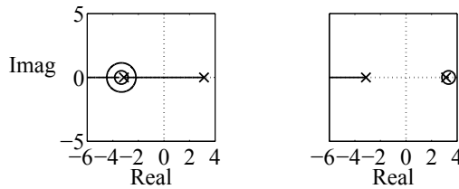
Abb. A.60: Wurzelortskurve für P-Regelung (links: Vorderradlenkung, rechts: Hinterradlenkung)
