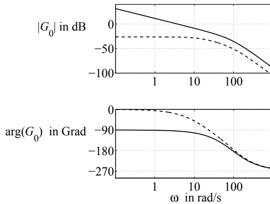
Abb. 11.23: Bodediagramm der offenen Kette bestehend aus Gleichstrommotor und PI-Regler
