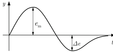
Abb. 11.6: Störverhalten des Regelkreises bei verzögerter Störung am Streckenausgang
