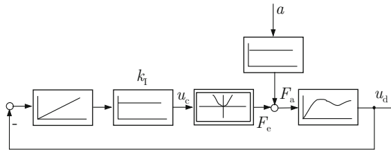
Abb. A4.4: Kompensationskreis des Airbag-Sensors
