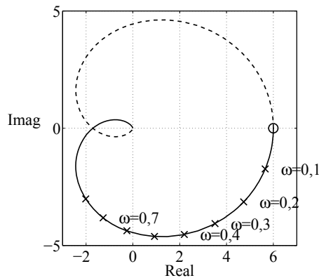
Abb. 6.9: Ortskurve mit Angabe ausgewählter Frequenzen
