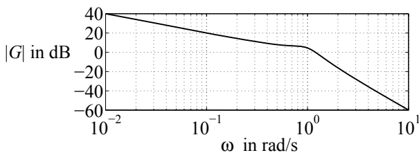
Abb. 6.55: Amplitudengang eines hydraulischen Ruderstellsystems
