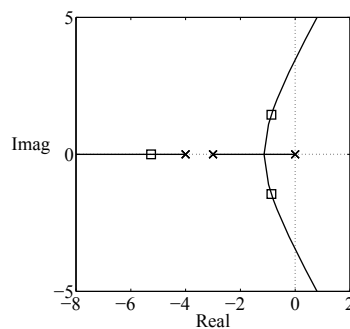
Abb. A.56: Wurzelortskurve mit dynamischem Regler (Pole \square für k = 15 )
