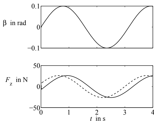
Abb. A.62: Lenkwinkel \beta und Kraftverlauf F_z bei Vorder- und Hinterradlenkung im Vergleich
