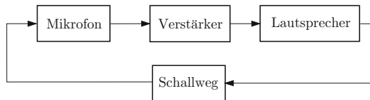
Abb. A.45: Blockschaltbild der Lautsprecheranlage
