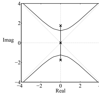
Abb. A.54: Wurzelortskurve der P-geregelten Verladebrücke
