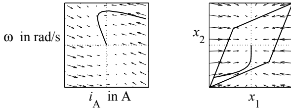
Abb. 5.13: Vektorfeld des Gleichstrommotors (links im i_A/\omega -Koordinatensystem; rechts im transformierten Zustandsraum \tilde{x}_1/\tilde{x}_2 )
