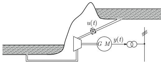
Abb. 6.60: Wasserkraftwerk
