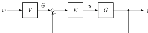
Abb. 7.8: Regelkreis mit Vorfilter
