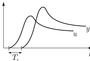
Abb. 5.41: Verhalten eines Totzeitgliedes
