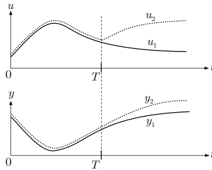
Abb. 4.5: Interpretation der Kausalität dynamischer Systeme
