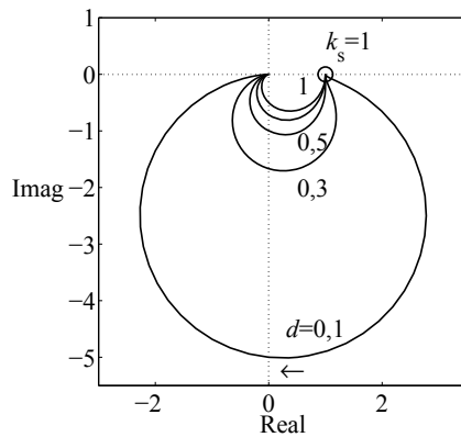
Abb. 6.42: Ortskurven von PT 2 -Gliedern mit k_s = 1 , T = 1 und d = 0,1, 0,3, 0,5, 0,7 und 1
