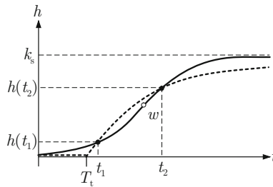
Abb. 5.50: Approximation einer Übergangsfunktion durch die Übergangsfunktion eines PT_t T_1 -Gliedes
