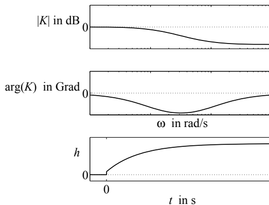
Abb. 7.32: Bodediagramm und Übergangsfunktion eines phasenabsenkenden Korrekturgliedes ( T = 10 s, T_D = 1 s)
