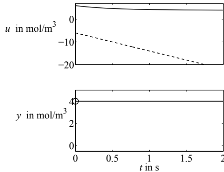
Abb. 6.64: Steuerung des minimalphasigen (—) und des nichtminimalphasigen Reaktors (- -)
