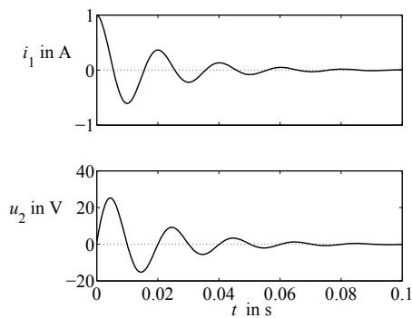
Abb. 4.11: Verlauf von Strom und Spannung des Reihenschwingkreises
