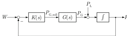
Abb. A.41: Blockschaltbild der Frequenzregelung
