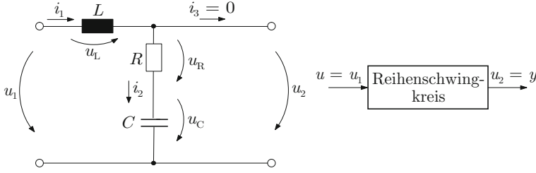
Abb. 4.2: Schaltung und Blockschaltbild eines Reihenschwingkreises
