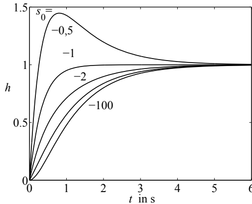
Abb. 6.48: Übergangsfunktion des Systems G(s, s_0) = -\frac{3}{s_0} \frac{s-s_0}{(s+1)(s+3)} für unterschiedliche Werte von s_0
