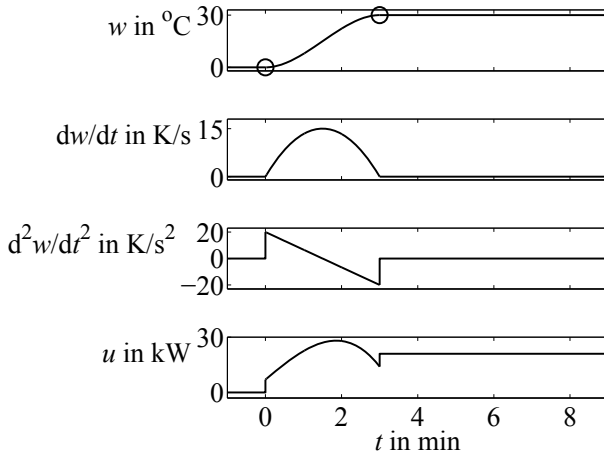
Abb. 7.27: Solltrajektorie w(t) , \dot{w}(t) und \ddot{w}(t) sowie Stellgröße u(t) für den Rührkesselreaktor bei t_e = 3 min
