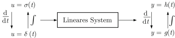
Abb. 5.20: Zusammenhang zwischen Gewichtsfunktion und Übergangsfunktion
