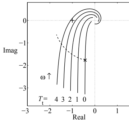
Abb. 8.14: Ortskurve einer I-Kette mit Totzeit T_t = 0 \dots 4
