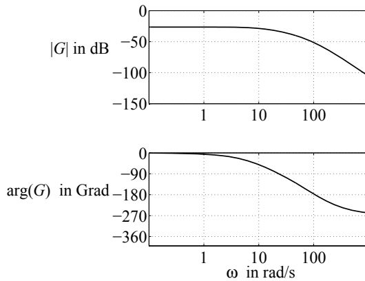
Abb. 11.22: Bodediagramm des Gleichstrommotors
