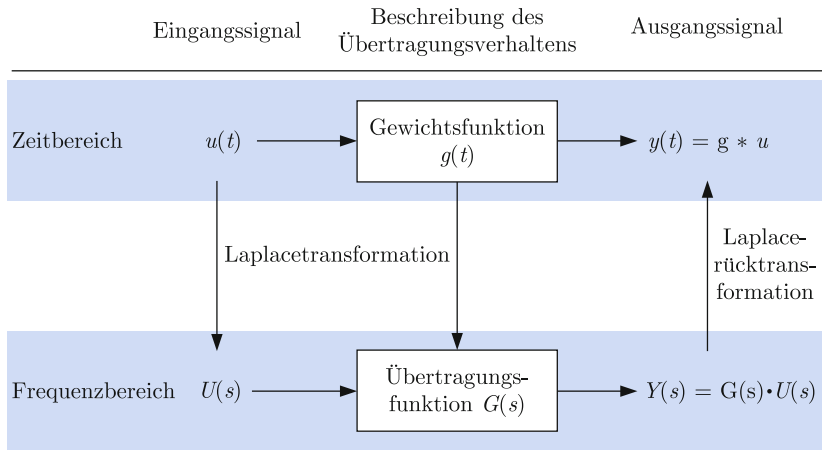
Abb. 6.21: Rechenschema für die Berechnung des Systemverhaltens mit Hilfe der Laplacetransformation
