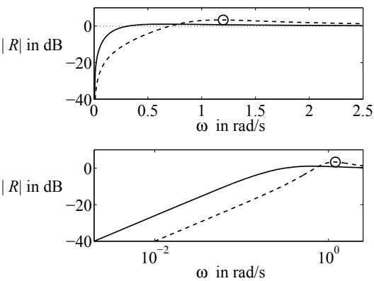
Abb. 7.15: Regelfaktor
