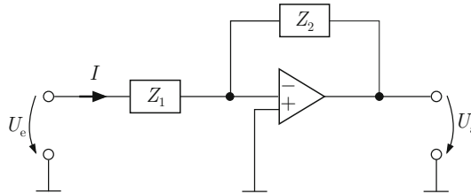
Abb. 7.34: Technische Realisierung von Reglern durch eine Operationsverstärkerschaltung
