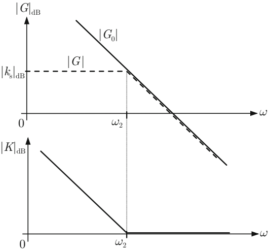
Abb. 11.13: Verbesserung des statischen Verhaltens durch Verwendung eines PI-Reglers
