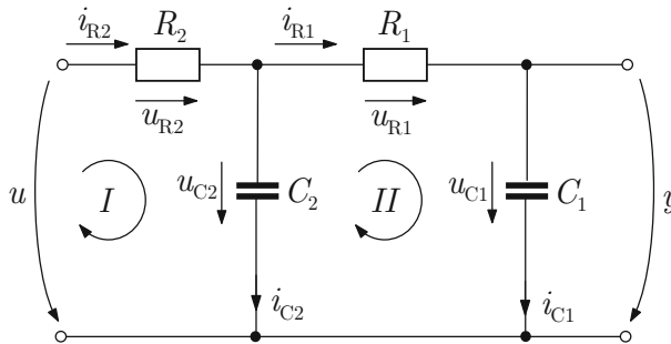
Abb. A.8: RC-Glied
