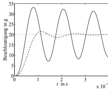
Abb. A.87: Messergebnis bei a(t) = 20g\sigma(t)
