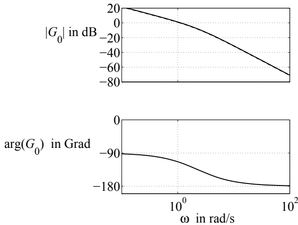
Abb. 11.18: Bodediagramm der offenen Kette mit PI-Regler
