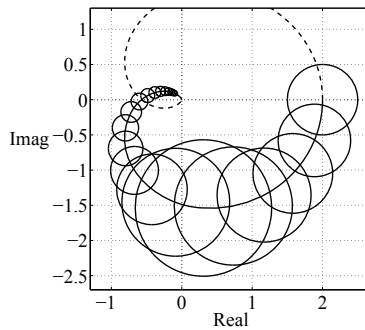
Abb. 8.24: Toleranzband für die Ortskurve eines Systems dritter Ordnung mit Modellunsicherheiten
