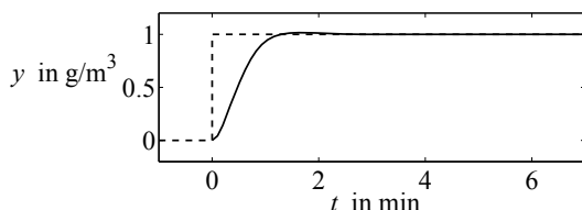
Abb. 12.12: Führungsübergangsfunktion des PI-geregelten Systems ohne Totzeit
