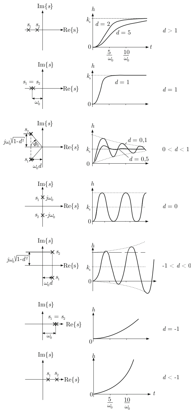
Abb. 6.32: Pole und Übergangsfunktion eines PT 2 -Gliedes
