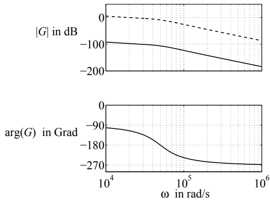
Abb. A.84: Frequenzkennlinien der offenen Kette
