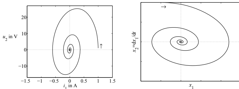
Abb. 4.12: Bewegung des Reihenschwingkreises im Zustandsraum (links) und Phasenporträt eines schwingenden Systems (rechts)
