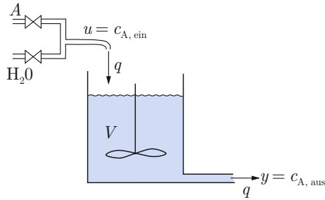
Abb. 6.71: Kontinuierlich durchflossener Reaktor
