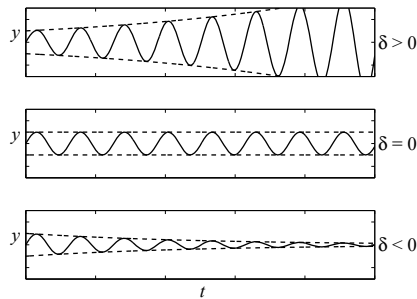
Abb. 6.12: Funktionen y(t) = e^{\delta t} \sin \omega t mit unterschiedlicher Dämpfung \delta
