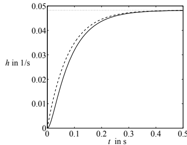
Abb. 5.45: Vergleich der Übergangsfunktionen des vollständigen — und des vereinfachten - - - Modells des Gleichstrommotors
