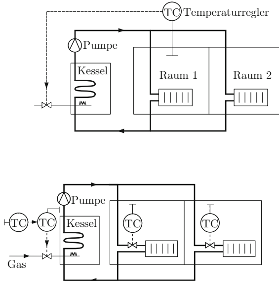
Abb. 2.1: Raumtemperaturregelungen
