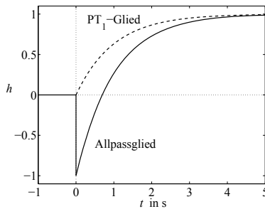
Abb. 6.57: Übergangsfunktion des Allpassgliedes G_A(s) = \frac{-Ts+1}{Ts+1} im Vergleich zu der des PT_1 -Gliedes \frac{1}{Ts+1} mit T = 1 s
