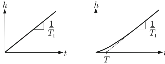
Abb. 5.36: Übergangsfunktion eines I-Gliedes (links) und eines IT_1 -Gliedes (rechts)
