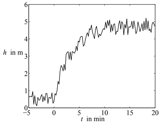
Abb. 5.48: Experimentell bestimmte Übergangsfunktion
