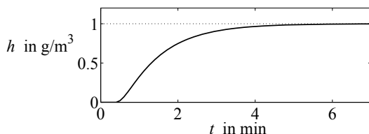
Abb. 12.11: Übergangsfunktion der Regelstrecke
