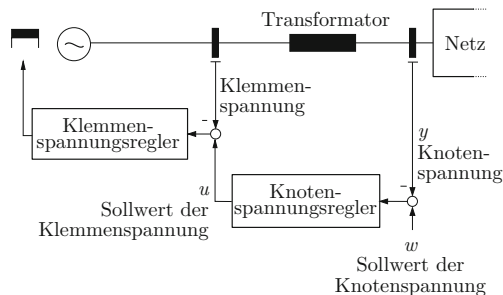
Abb. 11.16: Knotenspannungsregelung
