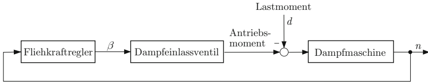
Abb. A.44: Regelkreis der Dampfmaschine
