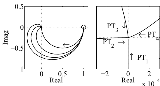
Abb. 6.44: Ortskurve von PT_n -Gliedern (Gesamtbild links und Ausschnitt um den Nullpunkt rechts)
