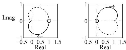
Abb. A.40: Ortskurve des Führungs- bzw. Störverhaltens des Regelkreises
