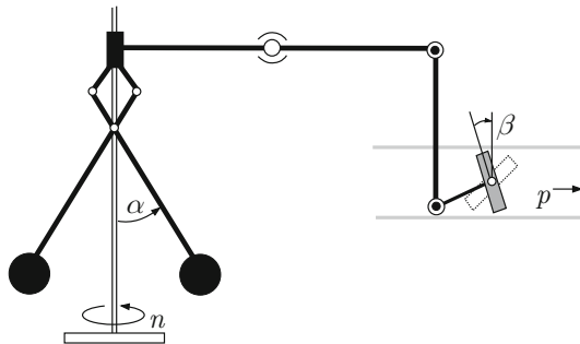
Abb. 1.4: Prinzip des Fliehkraftreglers
