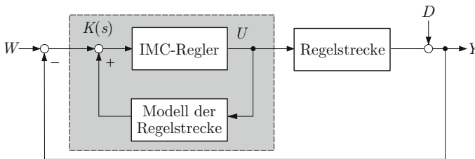
Abb. 12.5: Umgeformtes Blockschaltbild des IMC-Regelkreises
