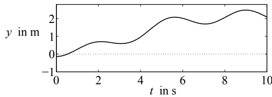
Abb. 5.8: Summe von Eigenbewegung und erzwungener Bewegung der Verladebrücke
