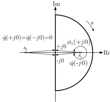
Abb. 8.6: Darstellung der Argumentänderungen für je einen Pol in der rechten und der linken komplexen Halbebene
