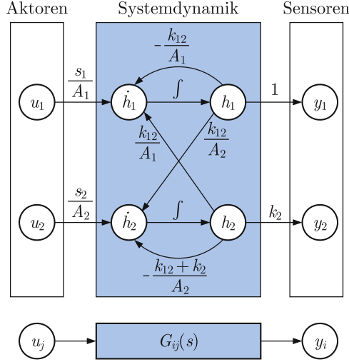
Abb. 6.19: Interpretation der Übertragungsfunktion des Behältersystems
