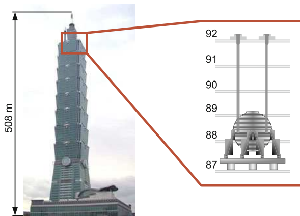
Abb. 6.74: Schwingungstilgung am Hochhaus
