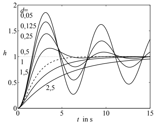
Abb. 6.34: Übergangsfunktionen eines Schwingungsgliedes mit T = 1 und k_s = 1
