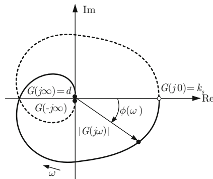
Abb. 6.8: Ortskurve eines nicht sprungfähigen Systems
