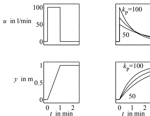
Abb. 1.9: Verhalten des Behälters bei einer Steuerung in der offenen Wirkungskette (links) und einer Regelung (rechts)
