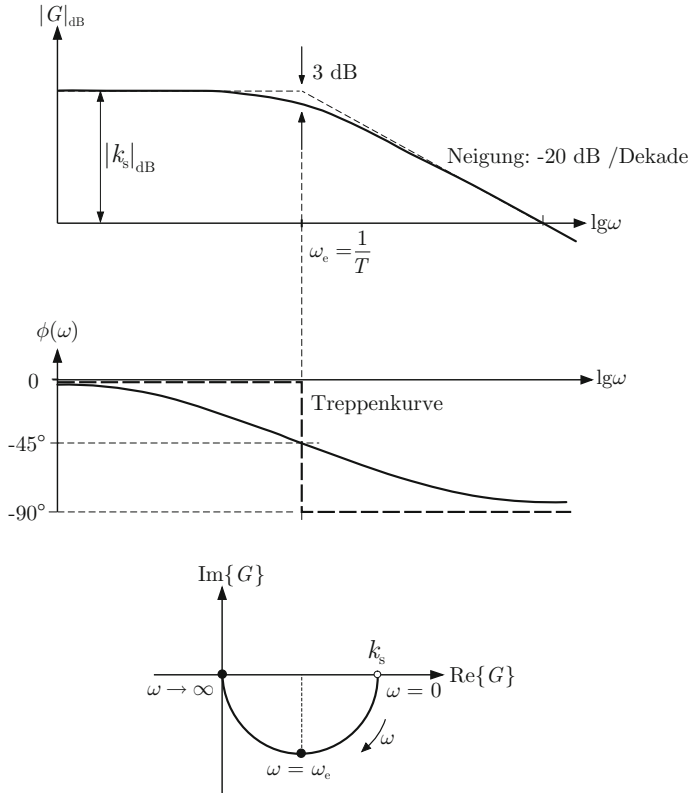
Abb. 6.30: Bodediagramm und Ortskurve eines PT_1 -Gliedes
