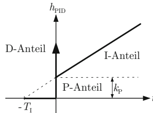
Abb. 7.31: Übergangsfunktion eines PID-Reglers
