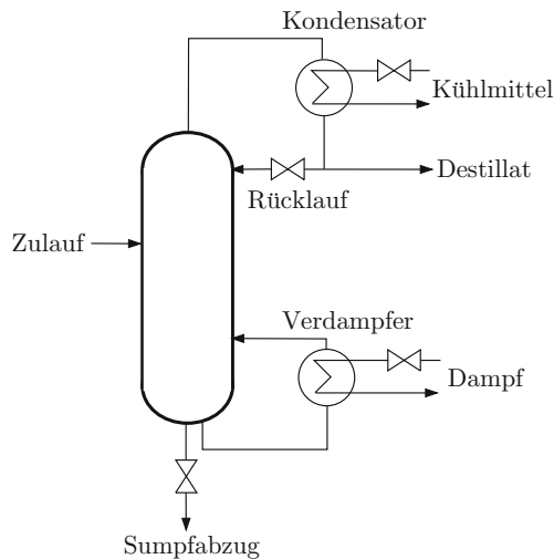
Abb. 2.4: Destillationskolonne
