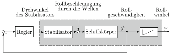
Abb. A.67: Blockschaltbild des Stabilisators
