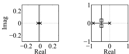
Abb. A.80: Wurzelortskurve mit P-Regler bzw. differenzierendem Korrekturglied
