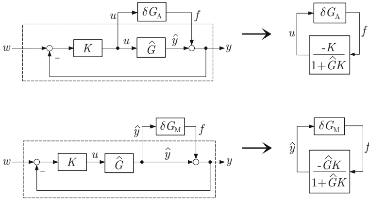
Abb. 8.19: Regelkreis mit additiver bzw. multiplikativer Modellunsicherheit
