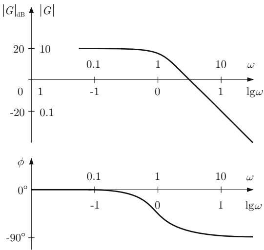
Abb. 6.10: Bodediagramm: Amplitudengang (oben) und Phasengang (unten) in logarithmischer Darstellung
