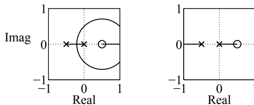
Abb. 10.14: Wurzelortskurve eines nichtminimalphasigen Systems
