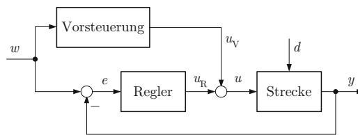
Abb. 1.7: Regelkreis mit zwei Freiheitsgraden
