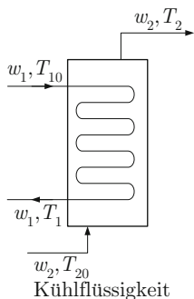
Abb. A4.2: Wärmeübertrager
