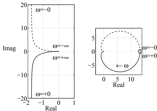
Abb. 8.13: Ortskurve einer I-Kette (links) und einer Kette mit Pol s_1 = -0,1 (rechts)
