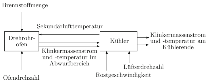
Abb. 3.4: Blockschaltbild zur Beschreibung der dynamischen Wechselwirkungen von Drehrohrofen und Klinkerkühler
