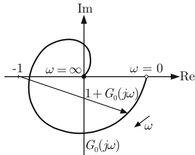
Abb. 7.13: Typischer Verlauf der Ortskurve der offenen Kette
