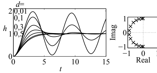
Abb. 6.38: Übergangsfunktionen von PT_2 -Gliedern mit unterschiedlicher Dämpfung d und derselben Eigenfrequenz \omega_0 = 1
