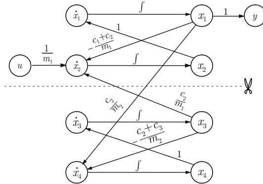
Abb. A.7: Signalflussgraph des Feder-Masse-Systems
