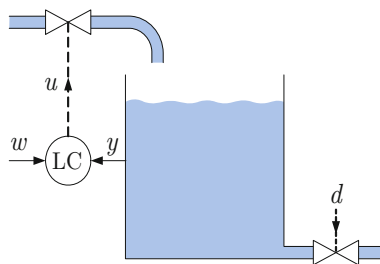
Abb. 1.8: Füllstandsregelung
