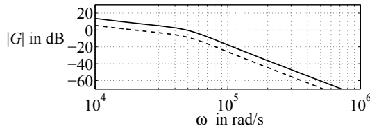
Abb. A.86: Verschiebung des Amplitudenganges der offenen Kette
