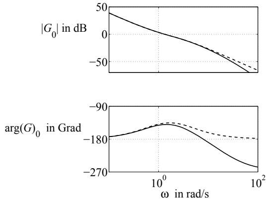
Abb. A.76: Bodediagramm der offenen Kette bei Berücksichtigung des Messgliedes
