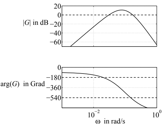
Abb. A.49: Bodediagramm der D-Kette
