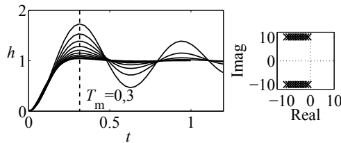
Abb. 10.4: Übergangsfunktion eines Schwingungsgliedes mit Polen bei \omega_e = 10 und \delta_e = 1, \dots, 10
