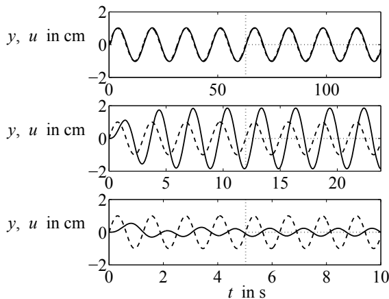
Abb. 6.7: Verhalten eines Feder-Masse-Schwingers bei sinusförmiger Erregung unterschiedlicher Frequenz
