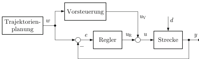
Abb. 7.21: Folgeregelung mit Trajektorienplanung und Vorsteuerung
