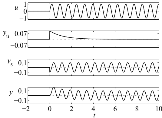
Abb. 5.22: Übergangverhalten und stationäres Verhalten eines Systems erster Ordnung
