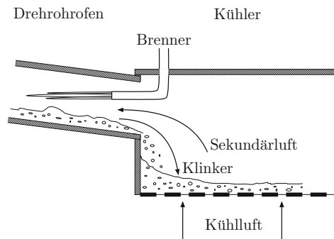
Abb. 3.3: Drehrohrofen und Klinkerkühler
