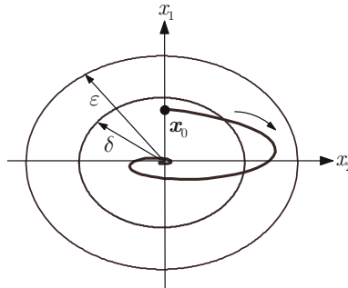
Abb. 8.1: Trajektorie eines asymptotisch stabilen Systems
