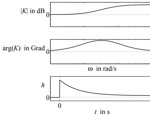
Abb. 7.33: Bodediagramm und Übergangsfunktion eines phasenhebenden Korrekturgliedes ( T_1 = 1 s, T_D = 10 s)
