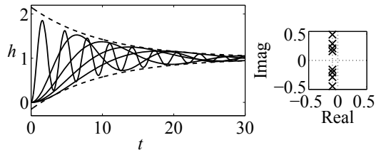
Abb. 6.35: Übergangsfunktion von PT_2 -Gliedern mit Polen \text{Re}\{s_i\} = -0,1
