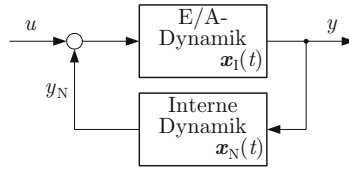
Abb. 5.16: Strukturbild des Zustandsraummodells in E/A-Normalform
