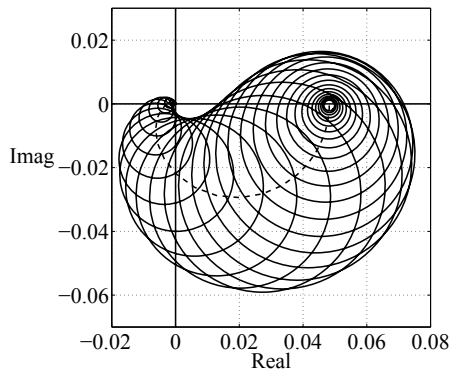
Abb. 8.21: Toleranzband für die Ortskurve des Gleichstrommotors
