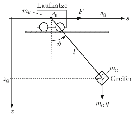
Abb. 5.5: Verladebrücke
