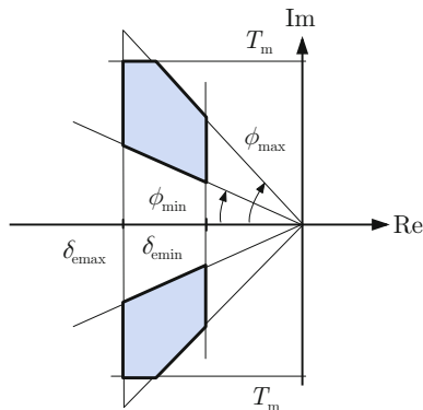
Abb. 10.8: Gebiete für die angestrebte Lage des dominierenden Polpaars des Regelkreises
