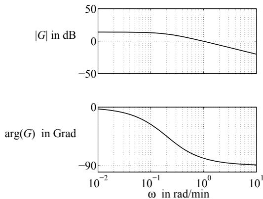
Abb. 6.72: Bodediagramm des Raumes
