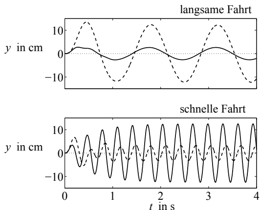
Abb. 7.18: Verhalten des Fahrzeugs bei sinusförmiger Störung (--- ohne aktive Dämpfung, — mit aktiver Dämpfung)
