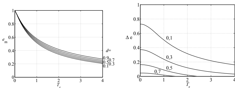
Abb. 11.9: e_m und \Delta e in Abhängigkeit von T_r = \frac{T_\Sigma}{T} und dem Parameter d
