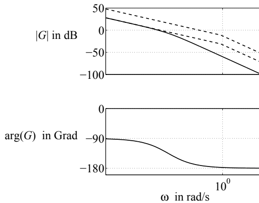
Abb. A.77: Bodediagramm der Regelstrecke und gewünschter Amplitudengang der offenen Kette
