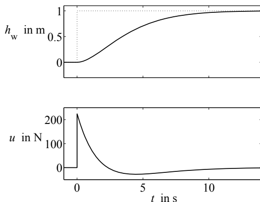
Abb. A.79: Führungsübergangsfunktion des Abstandsregelkreises
