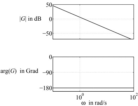
Abb. A.72: Bodediagramm des Flugzeugs als Regelstrecke
