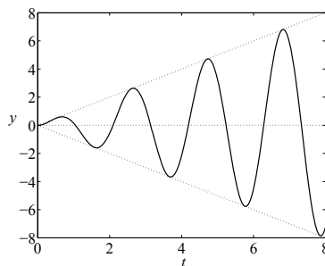
Abb. 5.23: Verhalten eines Oszillators bei Resonanz
