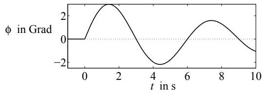
Abb. A.68: Rollbewegung des unregulierten Schiffes bei impulsförmiger Anregung
