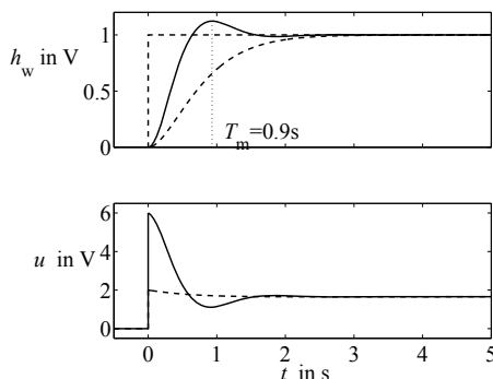
Abb. 11.21: Führungsübergangsfunktion des Regelkreises mit PI-Regler und Korrekturglied (---) sowie mit Korrekturglied und Verstärkungsanhebung (—)
