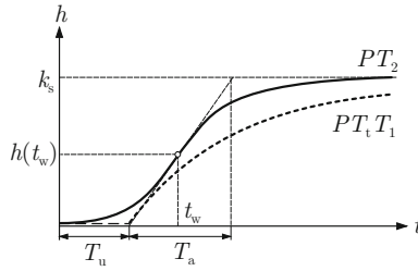
Abb. 5.49: Verzugszeit T_u und Anstiegszeit T_a der Übergangsfunktion von PT_2 -Gliedern
