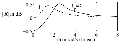
Abb. 7.17: Betrag des Regelfaktors R(j\omega) bei instabiler Regelstrecke
