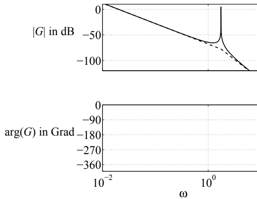
Abb. A.31: Bodediagramms der Verladebrücke
