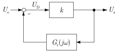
Abb. 6.28: Interpretation der Operationsverstärkerschaltung
