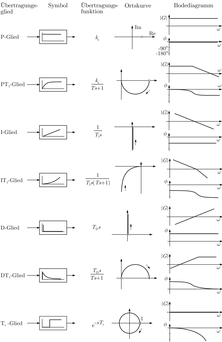
Abb. 6.53: Wichtige Übertragungsglieder
