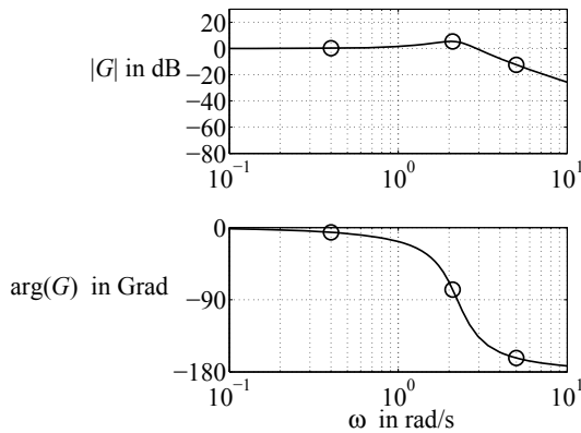
Abb. A.30: Bodediagramm des Feder-Masse-Schwingers
