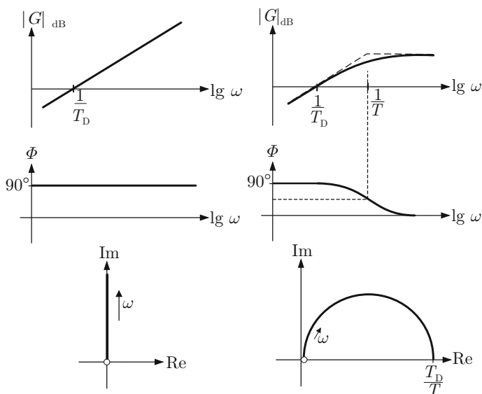
Abb. 6.47: Ortskurve und Bodediagramm eines D- und eines DT 1 -Gliedes
