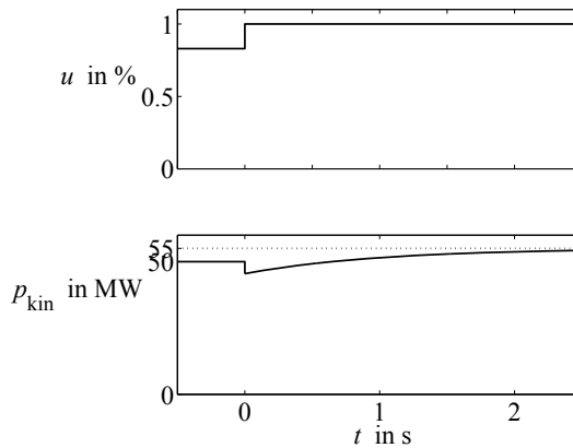
Abb. 6.61: Verhalten des Wasserkraftwerkes bei Leistungserhöhung von 50 MW auf 55 MW
