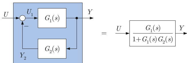
Abb. 6.24: Rückkopplungsschaltung zweier Übertragungsglieder
