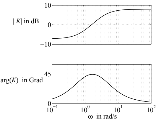
Abb. A.73: Bodediagramm des Reglers
