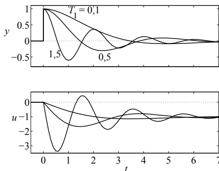
Abb. 7.11: Störübergangsfunktion eines Regelkreises mit I-Regler ( T_I = 0,1, 0,5 und 1,5 )
