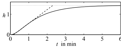
Abb. 9.2: Übergangsfunktion der Regelstrecke
