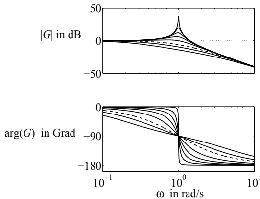
Abb. 6.39: Bodediagramm von PT_2 -Gliedern mit k_s = 1 , T = 1 und 0 < d < 1
