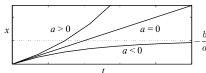
Abb. 5.2: Erzwungene Bewegung eines Systems erster Ordnung für sprungförmige Eingangsgröße (5.8)
