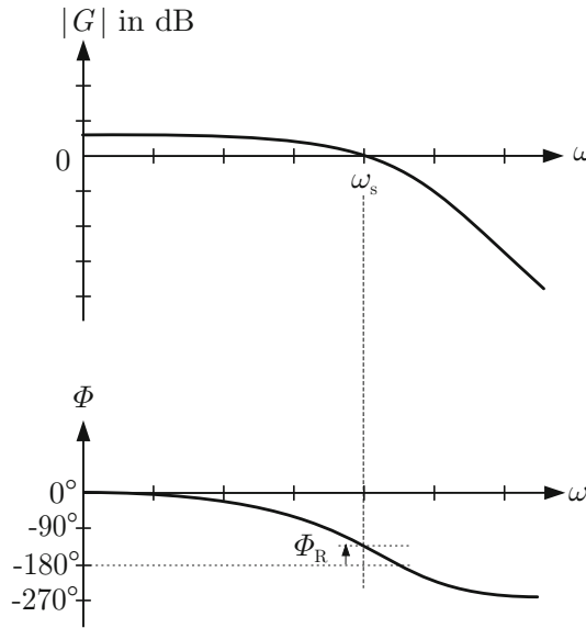
Abb. 8.17: Phasenrand im Bodediagramm
