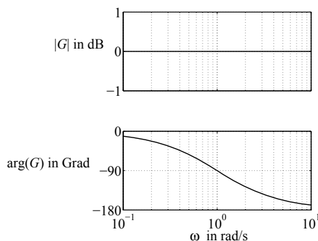
Abb. 6.56: Bodediagramm des Allpassgliedes (6.130) mit T = 1 s
