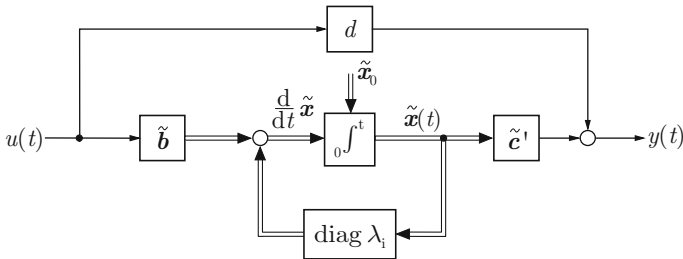
Abb. 5.10: Blockschaltbild des transformierten Modells
