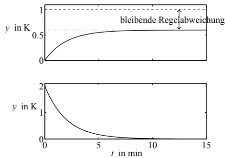
Abb. 5.52: Übergangsfunktion und Eigenbewegung des Raumtemperaturregelkreises
