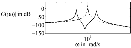
Abb. A.37: Vergleich des Amplitudenganges mit und ohne Dämpfer
