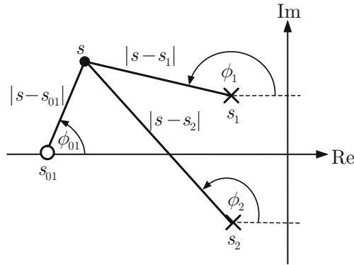
Abb. 10.10: Analyse der Wurzelortskurve
