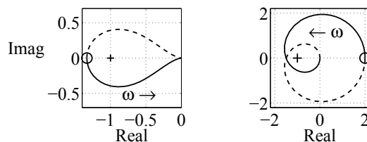
Abb. 8.10: Ortskurve zweier instabiler offener Ketten, die zu stabilen Regelkreises führen (links: ein instabiler Pol; rechts: zwei instabile Pole)
