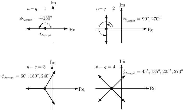
Abb. 10.12: Asymptoten der Wurzelortskurve für unterschiedlichen Polüberschuss der offenen Kette
