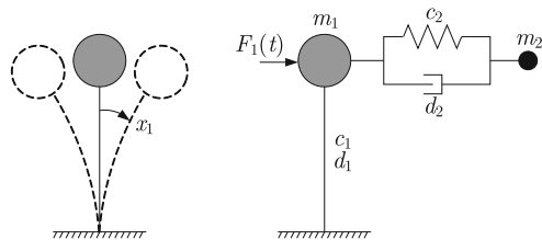
Abb. 6.75: Modellierungsansatz
