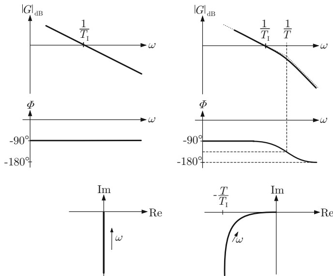
Abb. 6.46: Ortskurve und Bodediagramm eines I- und eines IT 1 -Gliedes
