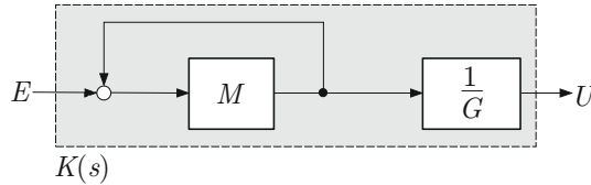
Abb. 12.2: Struktur des Kompensationsreglers
