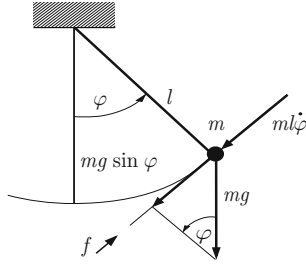
Abb. A.10: Kräftegleichgewicht am Pendel
