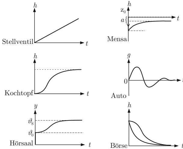
Abb. A.25: Qualitativer Verlauf der Übergangsfunktionen bzw. der Gewichtsfunction
