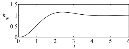
Abb. A.57: Führungsübergangsfunktion des Regelkreises
