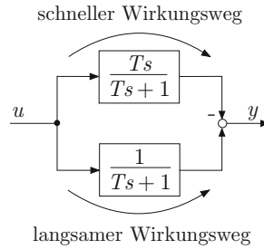
Abb. 6.58: Wirkung eines Allpassgliedes
