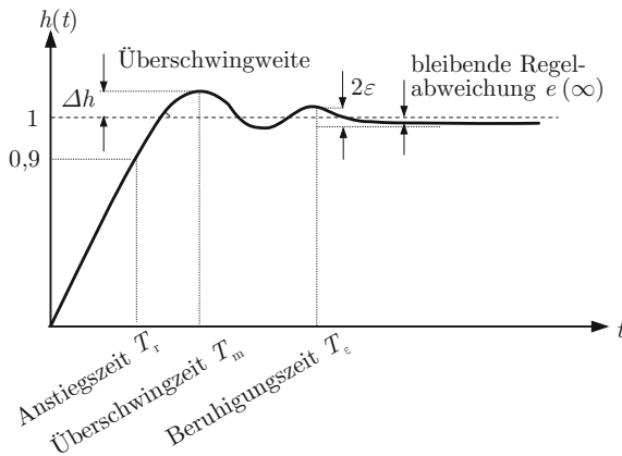
Abb. 7.1: Führungsübergangsfunktion des Regelkreises mit Kennzeichnung wichtiger Kennwerte
