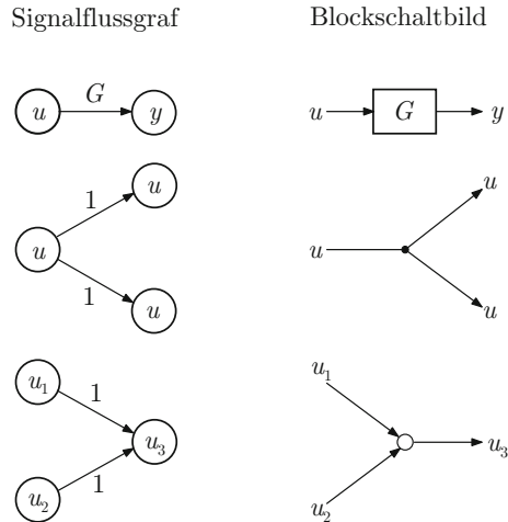
Abb. 3.12: Vergleich der wichtigsten Elemente von Signalflussgraphen und Blockschaltbildern
