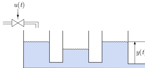
Abb. 4.22: 3-Tank-System
