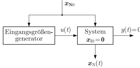
Abb. 5.27: Nulldynamik eines Systems
