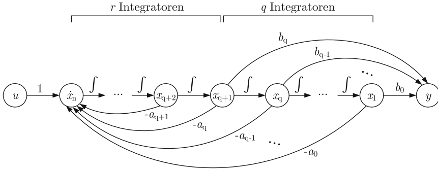
Abb. 4.16: Signalflussgraf für ein Zustandsraummodell in Regulationsnormalform ( 0 < r \leq n )
