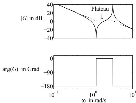
Abb. 6.51: Bodediagramm zur Übertragungsfunktion (6.124)
