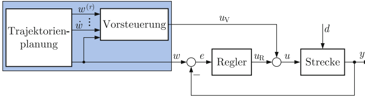
Abb. 7.24: Realisierung des Regelkreises mit Vorsteuerung und Trajektorienplanung
