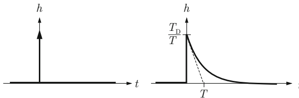
Abb. 5.40: Übergangsfunktion von D-Gliedern
