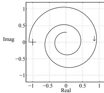
Abb. A.47: Ortskurve der Telefon-Radio-Anordnung für d = 0.3
