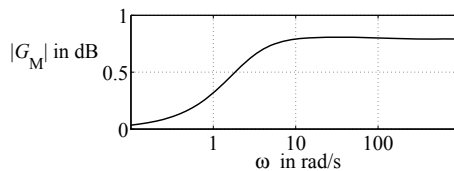
Abb. 8.22: Fehlerschranke \bar{G}_M(j\omega) für das Regelstreckenmodell
