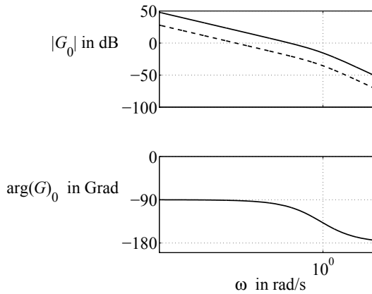
Abb. A.78: Bodediagramm der offenen Kette
