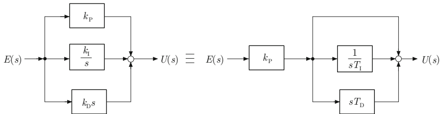
Abb. 7.30: Struktureller Aufbau eines PID-Reglers
