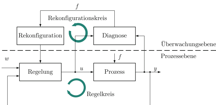
Abb. 13.6: Struktur fehlertoleranter Steuerungen
