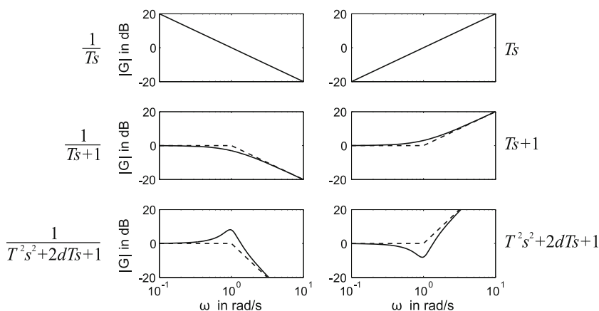
Abb. 6.49: Amplitudengang wichtiger elementarer Übertragungsglieder mit T = 1
