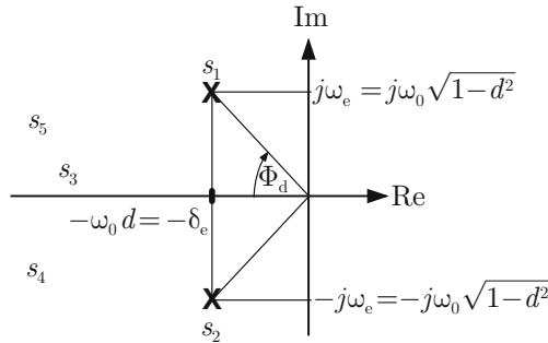
Abb. 10.2: PN-Bild eines Regelkreises mit dominierendem Polpaar
