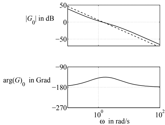
Abb. A.74: Bodediagramm der offenen Kette
