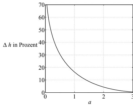
Abb. 11.3: Abhängigkeit der Überschwingweite \Delta h vom Einstellfaktor a
