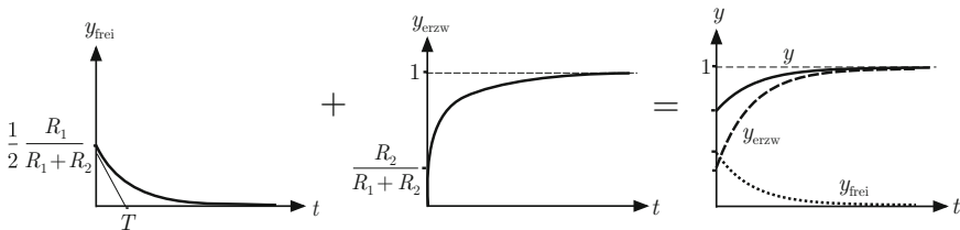
Abb. A.14: Überlagerung von Eigenbewegung und erzwungener Bewegung
