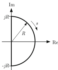
Abb. 8.4: Nyquistkurve \mathcal{D}
