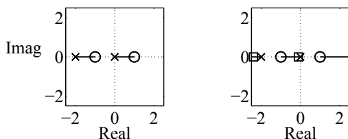
Abb. A.65: Wurzelortskurve für positive Reglerverstärkung k_P (links) und für negative Reglerverstärkung k_P (rechts; Pole \square für k_P = 0,2 )
