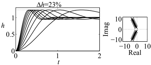
Abb. 10.6: Übergangsfunktion eines Schwingungsgliedes mit Polen auf den Dämpfungsgerade mit \phi_d = 65^\circ
