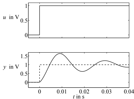
Abb. 7.28: Umsteuerung des Reihenschwingkreises mit konstanter Stellgröße
