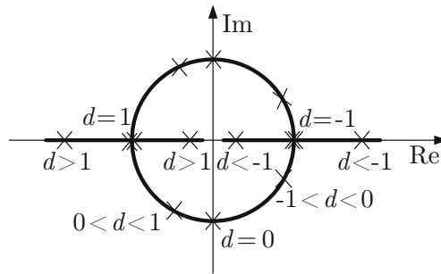
Abb. 6.37: Lage der beiden Pole von PT 2 -Gliedern in Abhängigkeit vom Dämpfungsfaktor d
