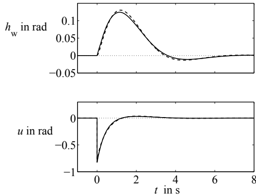
Abb. A.75: Störverhalten des Flugregelkreises
