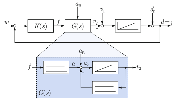
Abb. A.43: Regelung des Fahrzeugabstandes
