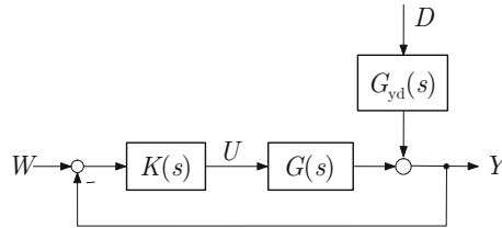
Abb. 11.7: Regelkreis mit der auf den Ausgang der Regelstrecke transformierten Störung
