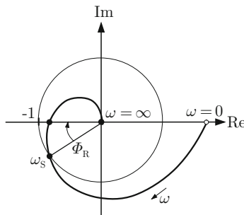
Abb. 8.16: Phasenrand einer Ortskurve
