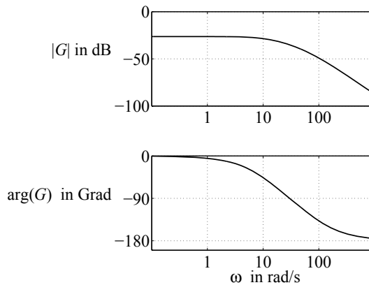
Abb. A.33: Bodediagramm des Gleichstrommotors
