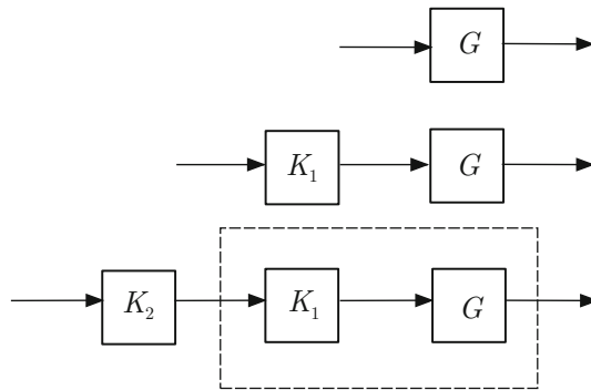
Abb. 11.10: Schrittweiser Entwurf des Reglers
