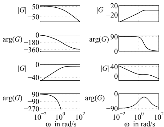
Abb. 6.70: Frequenzkennliniendiagramme von vier Systemen
