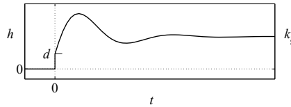
Abb. 5.17: Übergangsfunktion eines Systems zweiter Ordnung
