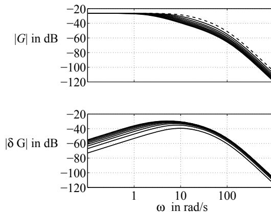
Abb. 8.20: Modell des Gleichstrommotors bei verändertem Trägheitsmoment J
