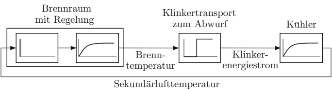
Abb. A.50: Vereinfachtes Blockschaltbild der Anordnung Drehrohrofen - Klinkerkühler
