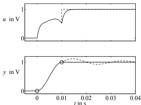
Abb. 7.29: Stationäres Verhalten bei veränderlicher und bei konstanter Stellgröße
