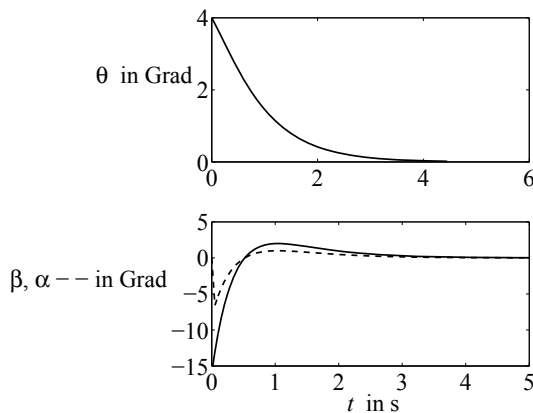
Abb. A.61: Verhalten des geregelten Fahrrades mit Vorderradlenkung
