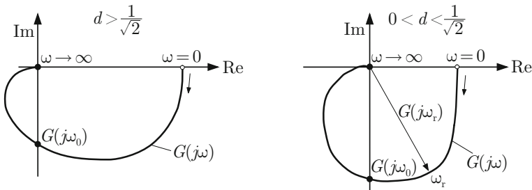
Abb. 6.41: Prinzipieller Verlauf der Ortskurve von PT 2 -Gliedern
