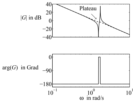
Abb. 6.52: Bodediagramm zur Übertragungsfunktion (6.125)
