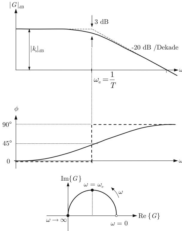
Abb. 6.31: Bodediagramm und Ortskurve eines instabilen Systems erster Ordnung
