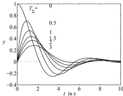
Abb. 11.8: Störübergangsfunktion bei verzögerter Störung ( d = 0,4 , T = 1 )
