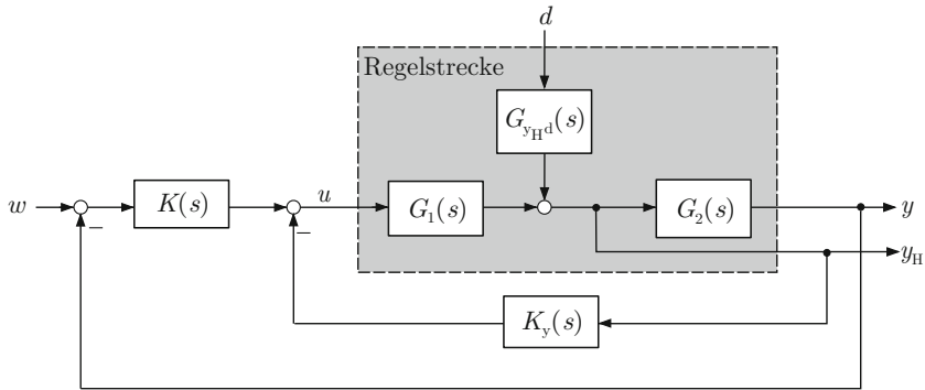
Abb. 13.3: Regelkreis mit Hilfsregelgröße
