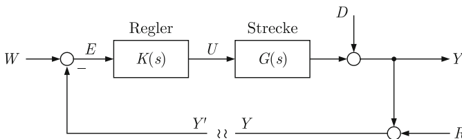
Abb. 7.4: Standardregelkreis
