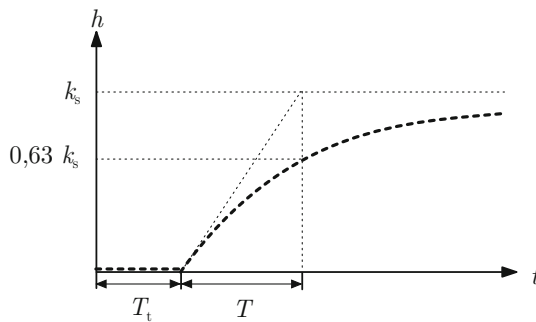
Abb. 9.1: Übergangsfunktion eines PT_1T_t -Gliedes
