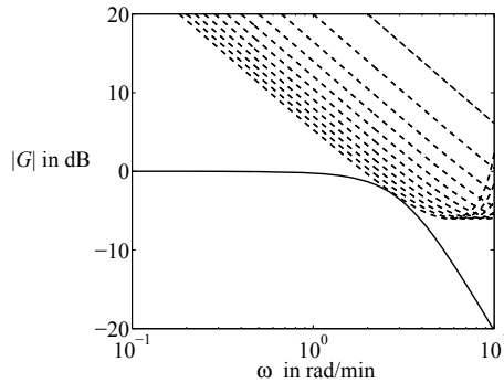
Abb. 12.18: Amplitudengang zur Überprüfung der robusten Stabilität des Smithprädiktor-Regelkreises
