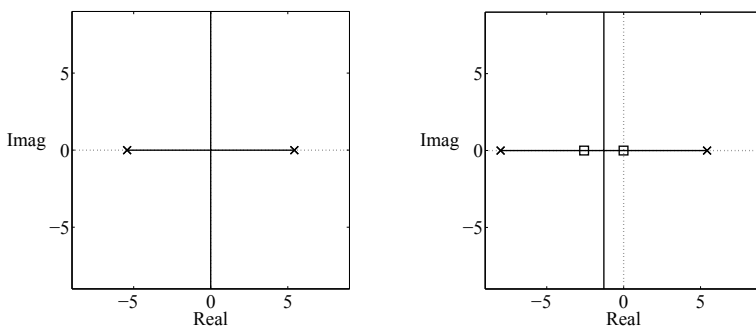
Abb. 10.17: Wurzelortskurve des Pendels mit P-Regler (links) und mit Korrekturglied (rechts) (Pole \square für die kritische Verstärkung)
