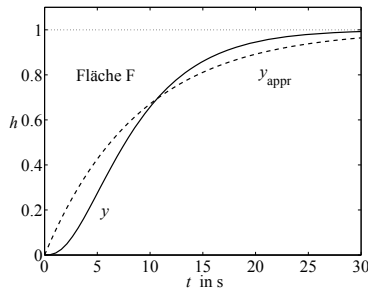
Abb. 5.46: Näherung eines PT_3 -Gliedes durch ein PT_1 -Glied mit derselben Summenzeitkonstante
