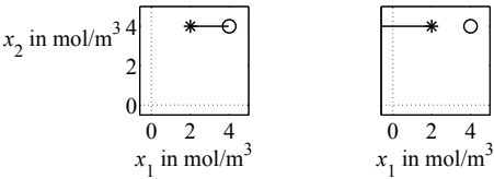
Abb. 6.65: Trajektorien des minimalphasigen (links) und des nichtminimalphasigen Reaktors (rechts) im Zustandsraum
