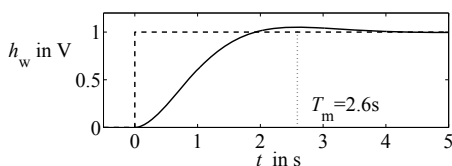
Abb. 11.19: Führungsübergangsfunktion des PI-geregelten Systems
