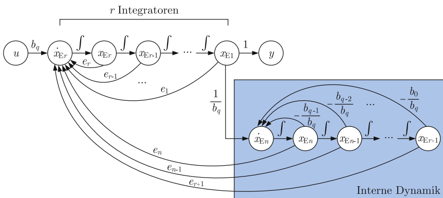
Abb. 5.15: Signalflussgraph des Zustandsraummodells in E/A-Normalform
