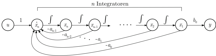
Abb. 4.15: Signalflussgraph für ein Zustandsraummodell mit Systemmatrix in Frobeniusform ( r = n )
