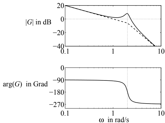
Abb. 6.50: Bodediagramm zur Übertragungsfunktion (6.123)
