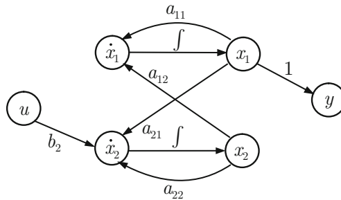
Abb. A.9: Signalflussgraf des RC-Gliedes
