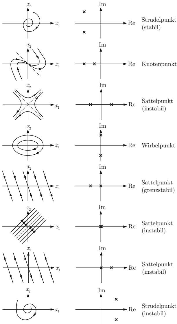
Abb. 8.2: Phasenporträts linearer Systeme zweiter Ordnung
