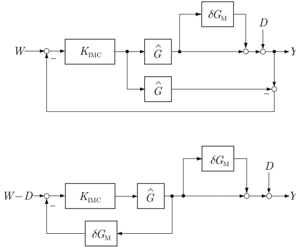
Abb. 12.7: Zwei äquivalente Darstellungen des IMC-Regelkreises mit Näherungsmodell
