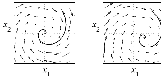
Abb. 4.10: Vektorfeld eines schwingungsfähigen Systems
