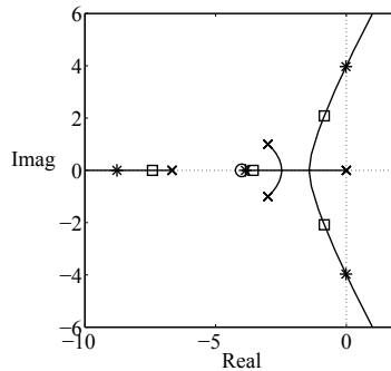
Abb. 10.9: Wurzelortskurve eines Regelkreises ( \square für k = 0,25 , * für k_{\text{krit}} = 2 )
