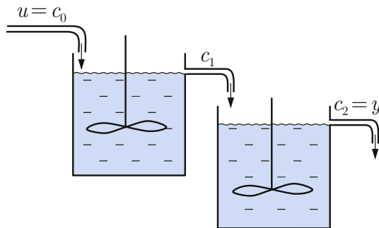
Abb. 5.9: Rührkessel
