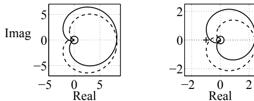
Abb. A.51: Ortskurve der Anordnung Drehrohrföfen – Klinkerkühler
