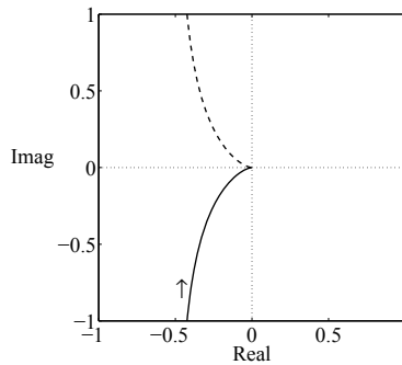
Abb. A.39: Ortskurve der offenen Kette
