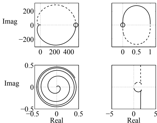
Abb. A.34: Ortskurven der vier Systeme
