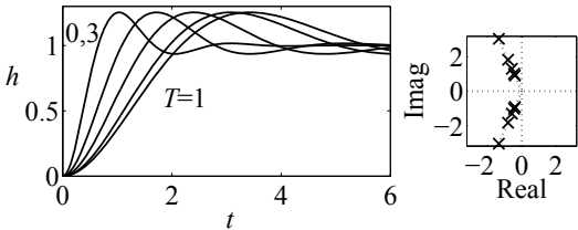
Abb. 6.36: Übergangsfunktion von PT 2 -Gliedern mit d = 0.4 und T = 0.3, 0.5, 0.7, 0.9 und 1
