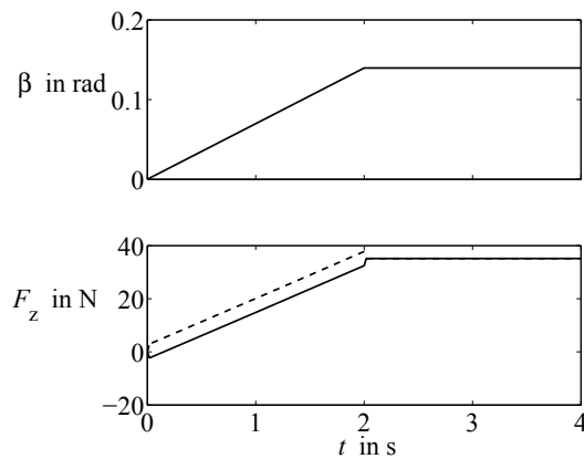
Abb. A.63: Lenkwinkel \beta und Kraftverlauf F_z bei rampenförmiger Lenkwinkelveränderung
