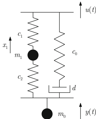
Abb. 5.24: Feder-Masse-Dämpfer-System
