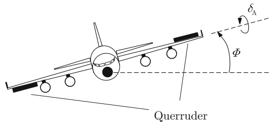
Abb. 5.14: Flugzeug als Regelstrecke
