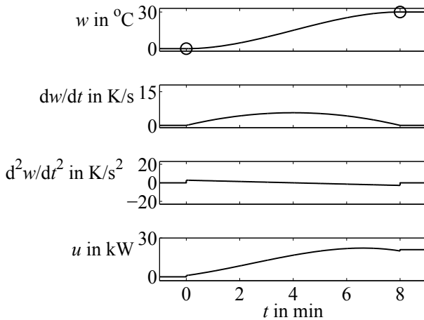
Abb. 7.26: Solltrajektorie w(t) , \dot{w}(t) und \ddot{w}(t) sowie Stellgröße u(t) für den Rührkesselreaktor bei t_e = 8 min
