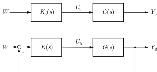
Abb. 7.20: Steuerkette und Regelkreis
