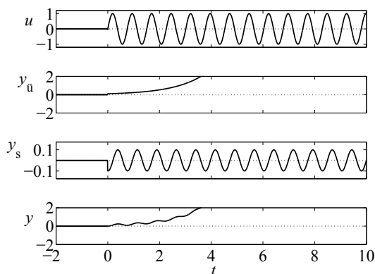
Abb. 6.14: Übergangsverhalten und stationäres Verhalten eines instabilen Systems erster Ordnung
