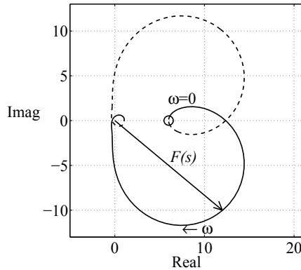
Abb. 8.5: Abbildung der Nyquistkurve durch die Rückföhrdifferenzfunktion F(s)
