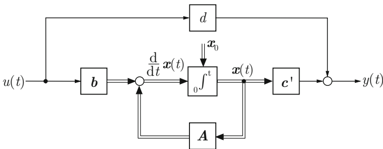
Abb. 4.7: Strukturbild des Zustandsraummodells
