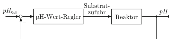
Abb. 3.6: Blockschaltbild der pH-Wert-Regelung
