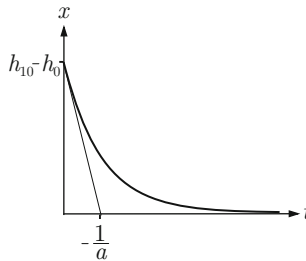
Abb. A.12: Eigenbewegung des Zweitanksystems
